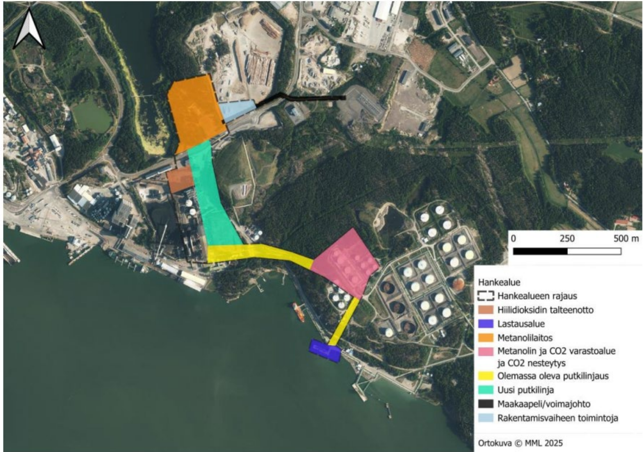
Kuva 1-3. Hankealue ilmakuvassa
